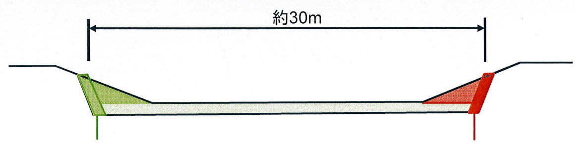
標準断面図
